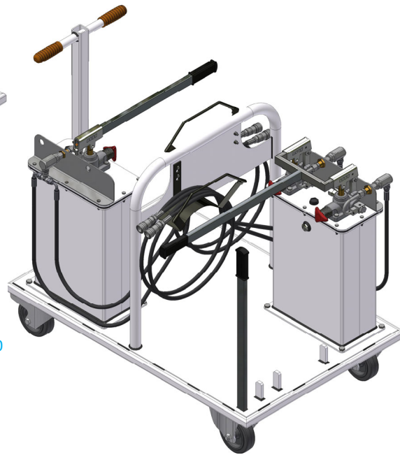
Separate unit TMH GA96-10-00 version Groupe séparé version TMH GA96-10-00
